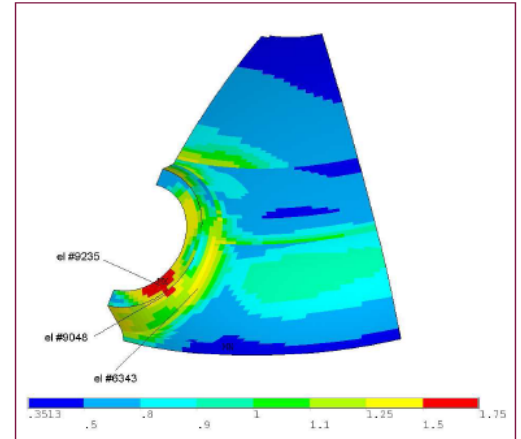
FEM-analyytikuvaa suodattimen miesluukun ympäristöstä
