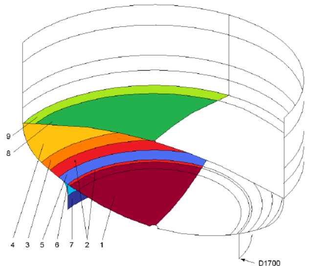
Laminaattirakenteiden paksuuksien määrittämistä mallitetulle suodattimen alaosalle
